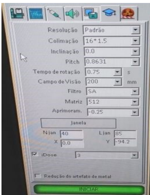
Figura 2 – Parâmetros técnicos do teste com simulador pediátrico
